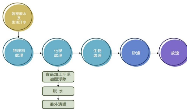
廢污水處理流程
